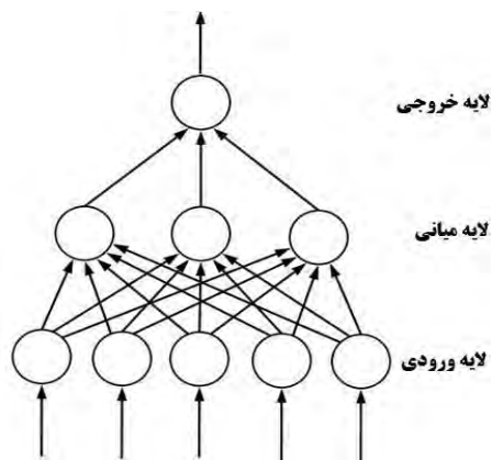
شکل (۱): نمای کلی شبکه عصبی پیشخور مورد استفاده در این مطالعه؛ در این مقاله مطابق روش استفاده شده به وسیله‌ی ژانگ (۱۹۹۸، ۲۰۰۳) و آلوداگ (۲۰۱۲) یک گره در لایه خروجی به کار رفته است. همچنین برای لایه ورودی نیز از دوازده گره استفاده شده است.
