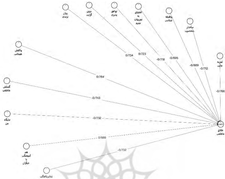
شکل ۱. مدل اندازه گیری در حالت در تخمین ضرایب استاندارد بدون حضور میانجی
