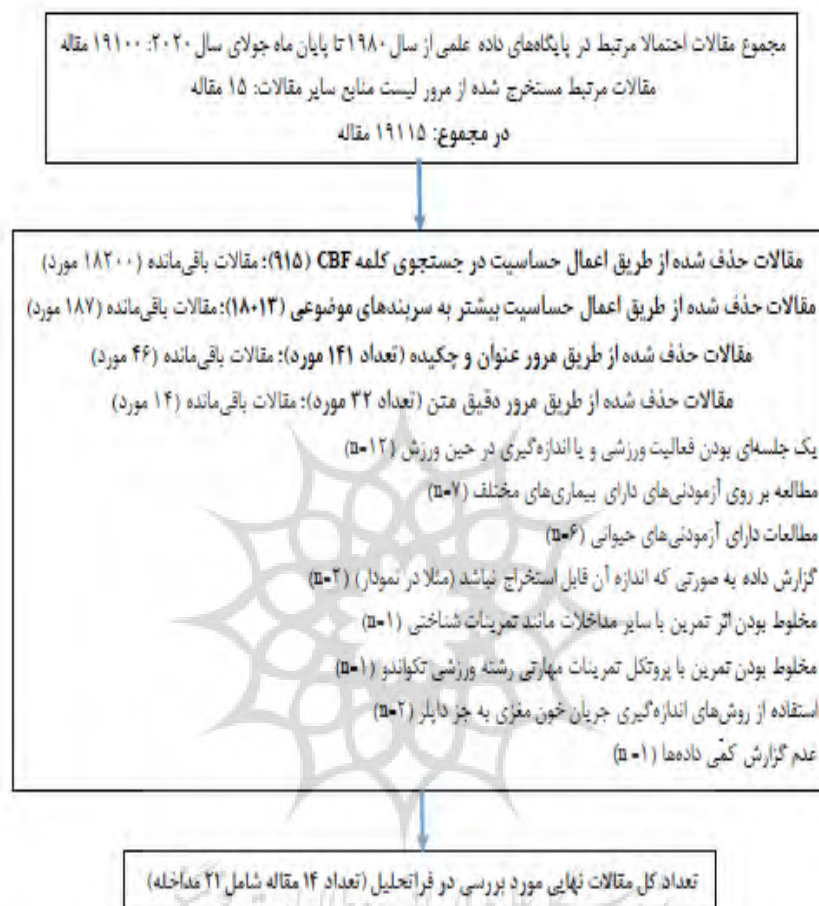
شکل ۱- طرح شماتیک اقدامات انجام شده برای انتخاب مقالات بررسی شده در فراتحلیل Fig1- Flow chart diagram of the study selection in meta-analysis
