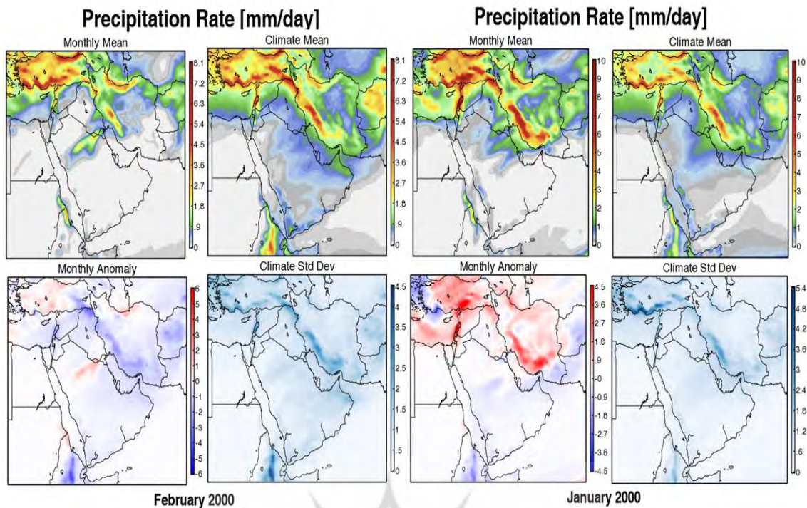
شکل ۷. از چپ به راست میانگین بارش، معدل اقلیمی، ناهنجاری بارش ماهانه، انحراف معیار خروجی MERRA-2 برای ماه ژانویه و فوریه ۲۰۰۰.
