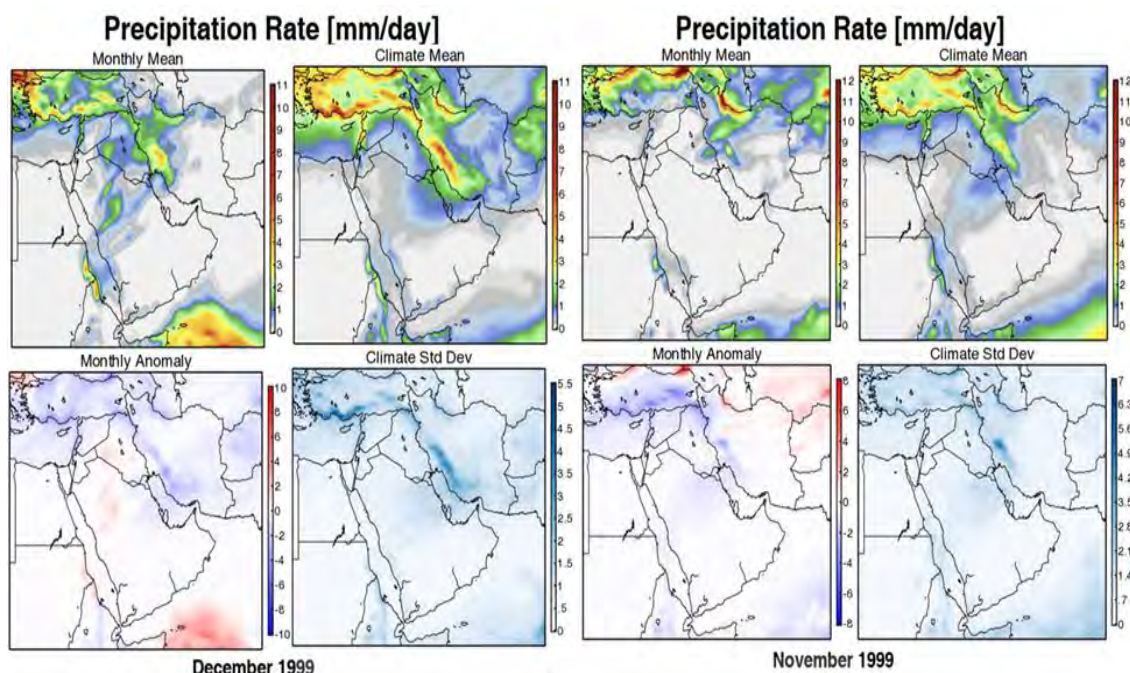
شکل ۶. از چپ به راست میانگین بارش، معدل اقلیمی، ناهنجاری بارش ماهانه، انحراف معیار خروجی MERRA-2 برای ماه نوامبر و دسامبر ۱۹۹۹.
