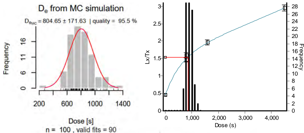
شکل ۹: نمودار مونت کارلو دانه های کوارتز نمونه RB1. سمت راست: در R و سمت چپ: در آنالیز برای ۱۰۰ تا برآورد
