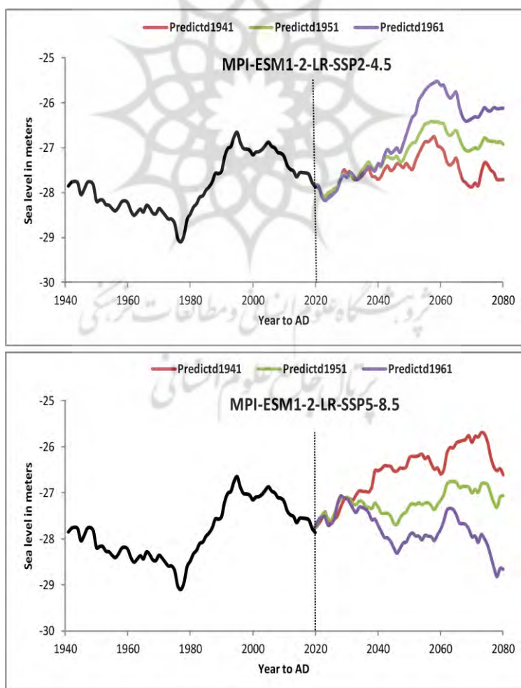
شکل شماره ۵. خروجی سناریوی SSP2-4.5 و SSP5-8.5 مدل اقلیمی MPI-ESM1-2-LR بر اساس دوره پایه ۶۰ تا ۸۰
