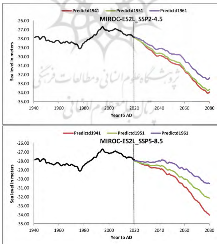
شکل شماره ۴. خروجی سناریوی SSP2-4.5 و SSP5-8.5 مدل اقلیمی MIROC-ES2L بر اساس دوره پایه ۶۰ تا ۸۰ ساله
