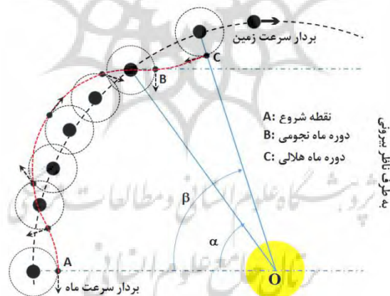
شکل ۱. دوره ماه نجومی B (۳۶۰ درجه دوران ماه از دید ناظر بیرونی) و دوره ماه هلالی یا اقترانی C (رویت ماه در نقطه در همان نقطه شروع از دید ناظر زمینی)
