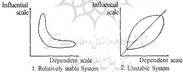
شکل ۲- پراکندگی مکانی متغیرها در سیستم‌های پایدار و ناپایدار (گوده - ۱۹۹۴)
