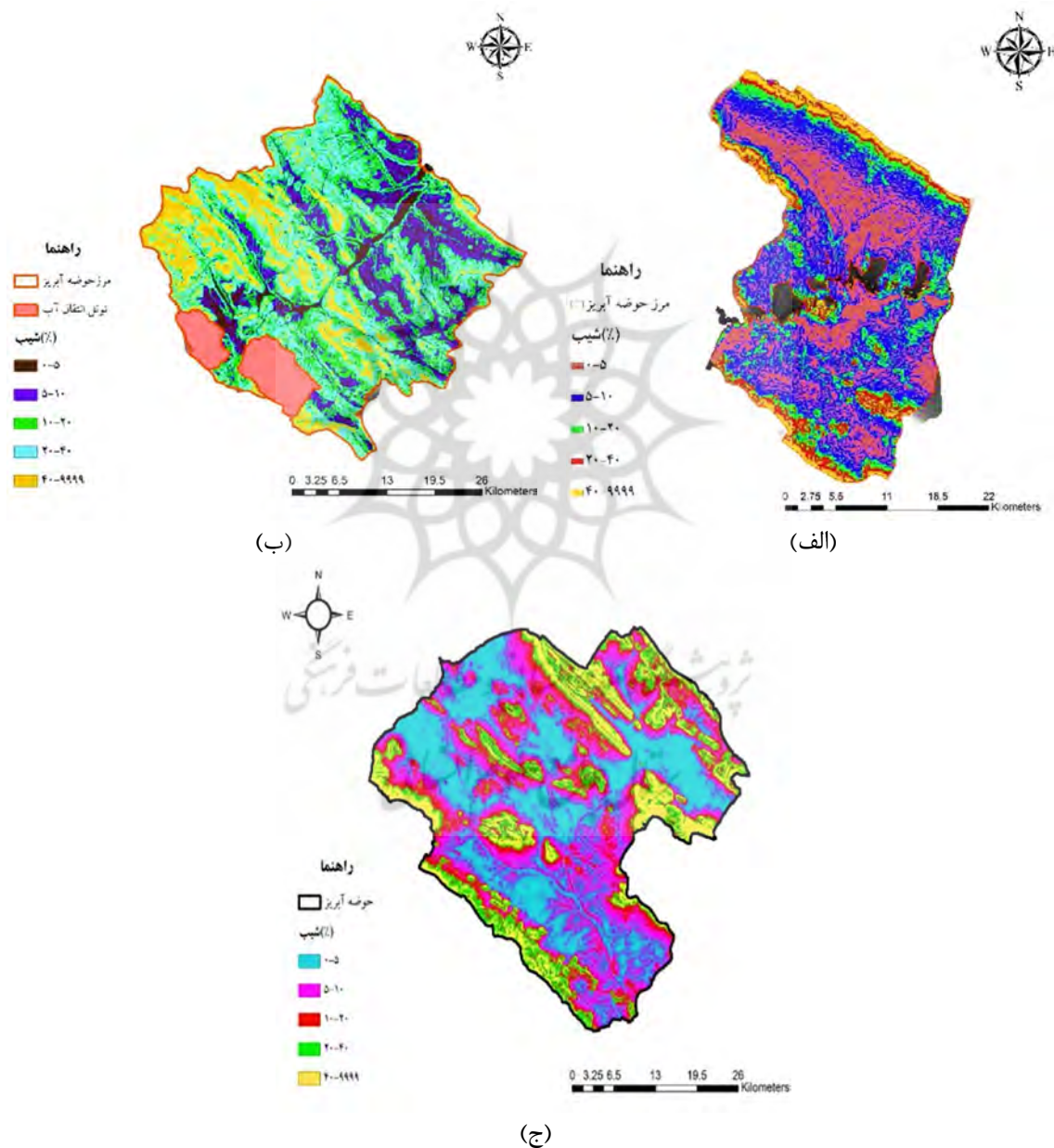
شکل ۶- نقشه شیب بندی در محیط GIS محور SWAT، زیر حوضه آبریز چادگان-بان چشمه (الف)، زیر حوضه آبریز قلعه شاهرخ-چلگرد (ب)، زیر حوضه آبریز دامنه-بوئین (ج)
