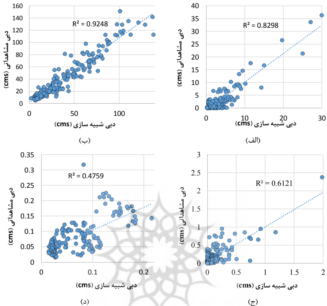
شکل ۸- نمودار پراکندگی داده‌های دبی مشاهده‌ای و دبی شبیه‌سازی شده در الف: ایستگاه اسکندری، ب: زیر حوضه قلعه شاهرخ-چلگرد، ج: ایستگاه مندرجان، د: ایستگاه حیدری
