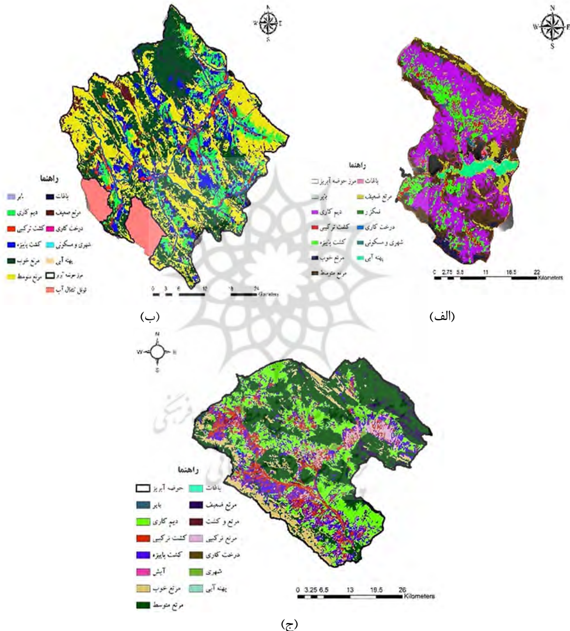
شکل ۴- نقشه کاربری اراضی زیر حوضه آبریز چادگان-یان چشمه (الف)، زیر حوضه آبریز قلعه شاهرخ-چلگرد (ب)، زیر حوضه آبریز دامنه-بوئین (ج)
