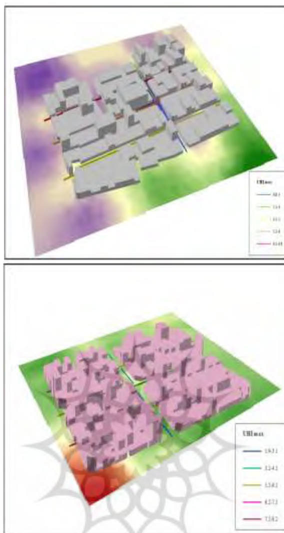
شکل‌های ۱۱ و ۱۲. به ترتیب از راست به چپ نمایش سه‌بعدی نتایج حاصل از شبیه‌سازی کوی ولیعصر و شنب‌غازان در
