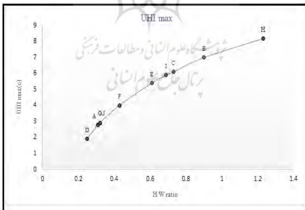
شکل ۹. ارتباط بین شدت UHI شبیه‌سازی شده و نسبت H/W کوی ولیعصر
