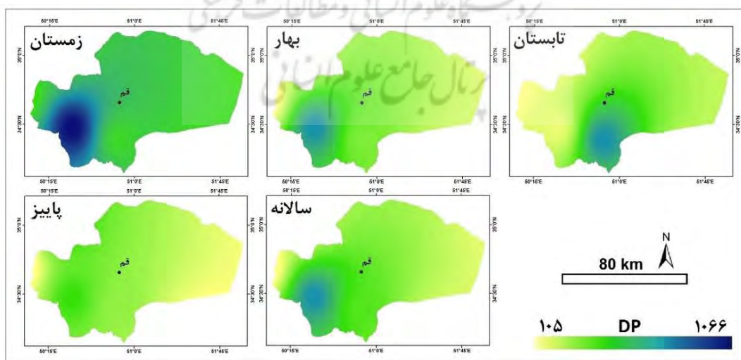
شکل ۷: نقشه‌های دورنیایی DP فصلی و سالانه استان قم
