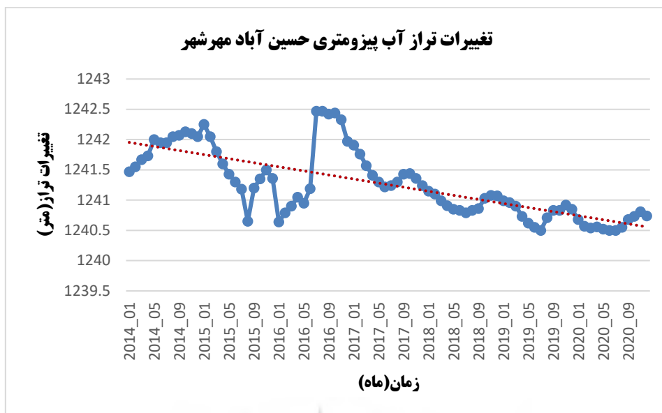
شکل (۷ج): نمودار تغییرات تراز آب پیرومتری حسین آباد مهرشهر در بازه زمانی ۲۰۱۴ تا ۲۰۲۰ بر حسب متر
