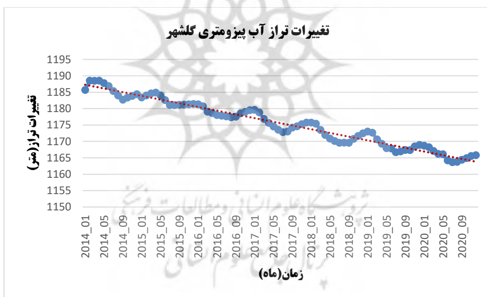
شکل (۷د): نمودار تغییرات تراز آب پیرومتری گلشهر در بازه زمانی ۲۰۱۴ تا ۲۰۲۰ بر حسب متر
