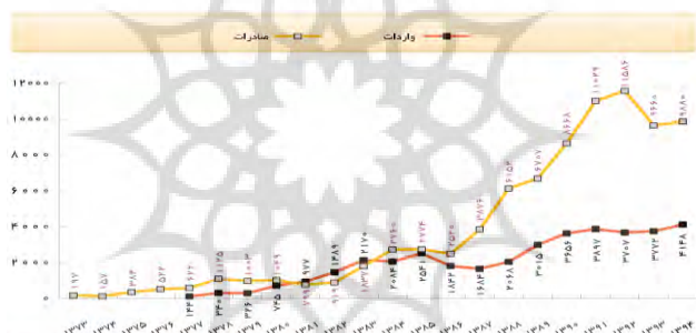
شکل ۱. حجم صادرات و واردات برق ایران از سال ۱۳۷۳ تا ۱۳۹۴ (بر حسب میلیون کیلووات ساعت)
