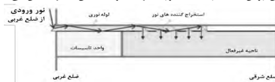
شکل ۵- برش عرضی لوله نوری افقی
