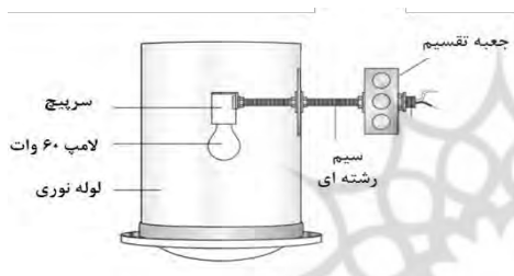
شکل ۱۷- لوله نوری به همراه کیت نور
