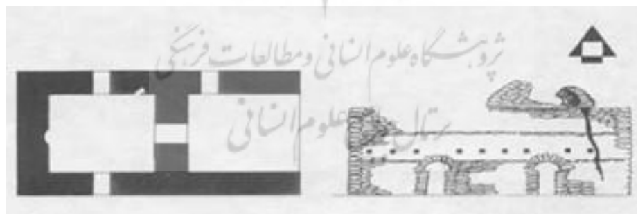
شکل ۹: نما و برش از قلعه هزار درب (میراث فرهنگی ایلام)
