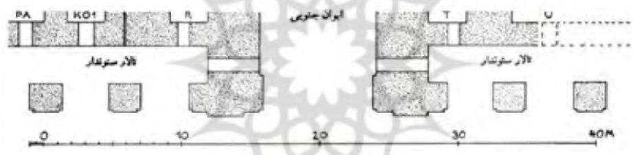
شکل ۸: نقشه سازه ای قلعه هزار درب (میراث فرهنگی ایلام)
