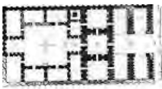
شکل ۵: پلان قلعه هزار درب (میراث فرهنگی ایلام)
