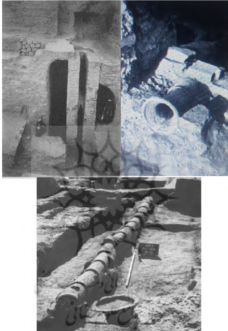
تصویر ۲: آبراهه نیایشگاه خدای بعل در اشنون (بالا، راست) (Antoniou, 2016: 4, Fig. 1.b)؛ آبراهه نیایشگاه همین خدا در نیپور (بالا، چپ) (Hilprecht, 1904: 40, Fig. 31)؛ لوله‌هایی از جنس گل پخته‌شده (هزاره چهارم) در چغامیش (پایین) (Antoniou, 2016: 4, Fig. 1.a)
