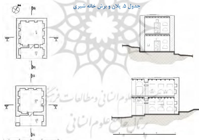
جدول ۵. پلان و برش خانه شیری
