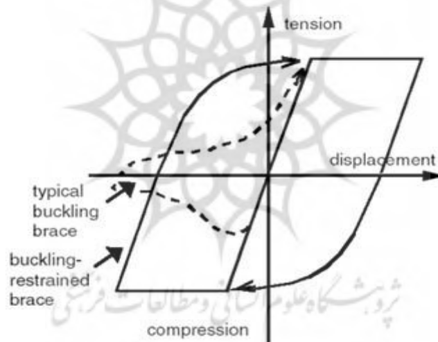
شکل ۱- گام های مختلف اعمال بار، در بارگذاری سیکلی یک مهاربند در صورتی که از کمانش عضو در فشار جلوگیری شود، حلقه‌ی هیستریزس به شکل زیر خواهد بود.
