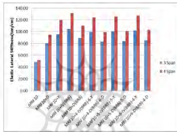
شکل ۶-مقایسه سختی سازه های ۱۰ طبقه
