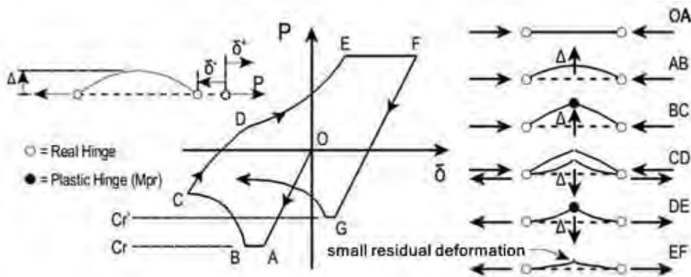
شکل ۱- گام های مختلف اعمال بار، در بارگذاری سیکلی یک مهاربند در صورتی که از کمانش عضو در فشار جلوگیری شود، حلقه‌ی هیستریزس به شکل زیر خواهد بود.
