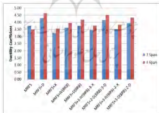
شکل ۷-مقایسه شکل پذیری سازه های ۵ طبقه
