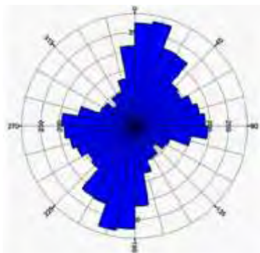
شکل ۷. رزدياگرام خطواره‌های موجود در توده آهکی دوساری
