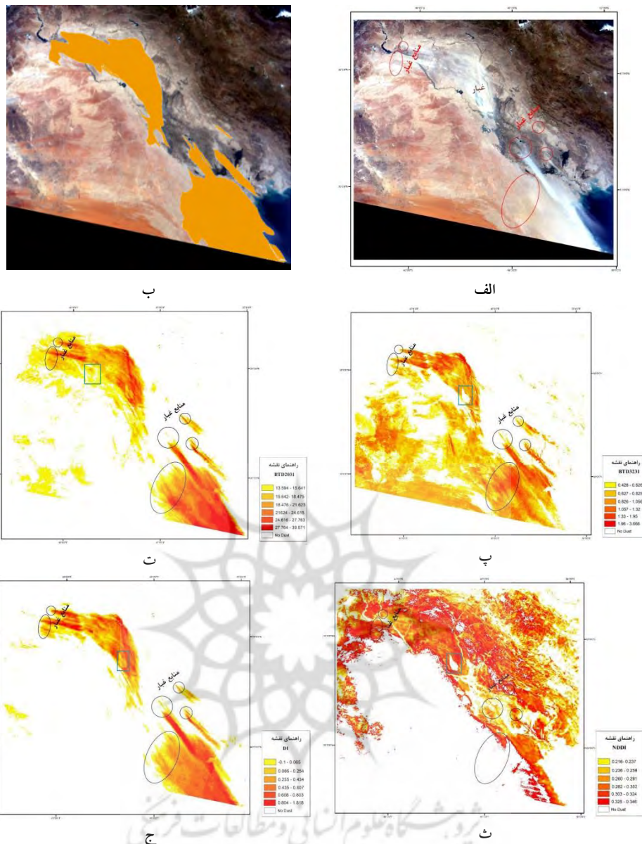
شکل ۴- الف) تصویر رنگی مادیس، ب) طوفان غبار بدست آمده بر روی تصویر رنگی مادیس و مقایسه‌ی نتایج اعمال پ) BTD_{32-31} ، ت) BTD_{20-31} ، ث) NDDI و ج) DI بر روی رخداد طوفان غبار در ۲۷ خرداد ماه ۱۳۸۷ با در نظر گرفتن حدآستانه‌های مناسب.
