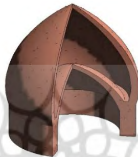
تصویر ۲- مدل‌سازی گنبد مسجد امام اصفهان، نحوه‌ی اجرای گنبد حول محور عمودی،
