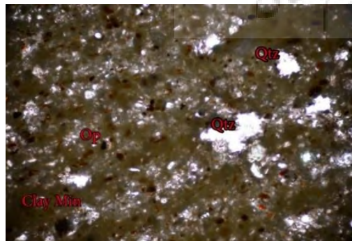
شکل ۲۴: وجود کانی اپک و کوارتز، بزرگنمایی ۱۰۰ حالت PPL Figure 24: the presence of Mineral Op & Quartz, 100x, PPL mode
