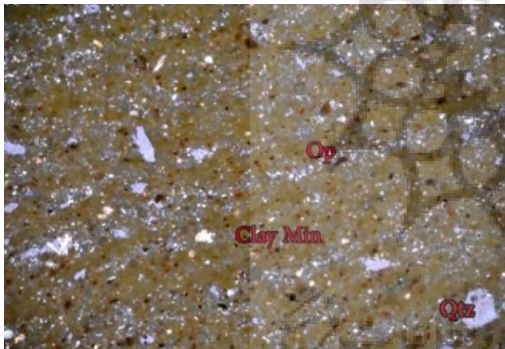
شکل ۲۲: وجود کانی رسی و کوارتز، بزرگنمایی ۴۰ حالت XPL Figure 22: the presence of quartz and clay minerals, 40x, XPL mode
