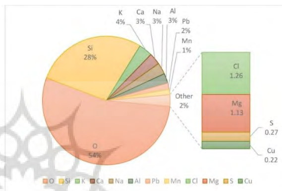
شکل ۶: نمودار میزان فراوانی درصد وزنی عناصر لعاب مشکی Fig. 6: Graph of the frequency percentage by weight of black glaze elements
