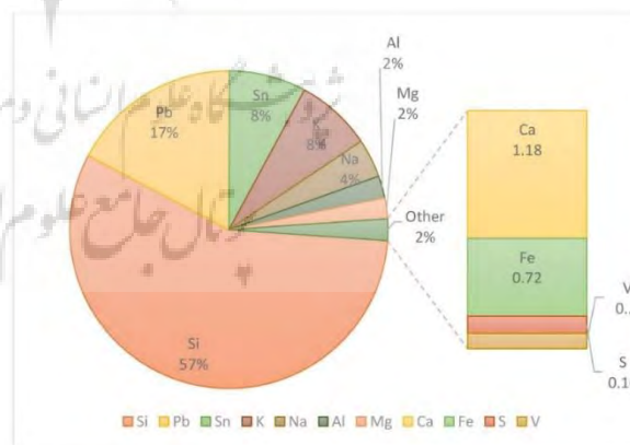
شکل ۷: نمودار میزان فراوانی درصد وزنی عناصر لعاب سفید Fig. 7: Graph of frequency percentage by weight of white glaze elements
