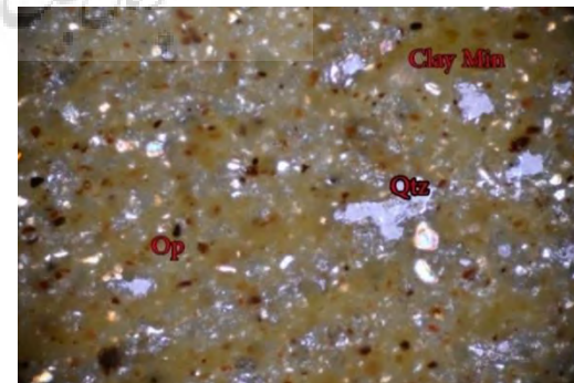
شکل ۲۳: کانی رسی، اپک و کوارتز، بزرگنمایی ۱۰۰ حالت XPL Figure 23: clay minerals, Op, Quartz, 100x, XPL mode
