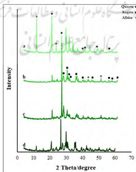
شکل ۲۹: الگوی XRD بدنه کاشی‌های (a) G-4، (b) B-4، (c) B-2 و (d) BL. Figure 29: XRD pattern of tile body a) G-4, b) B-4, c) B-2 and d) BL.
