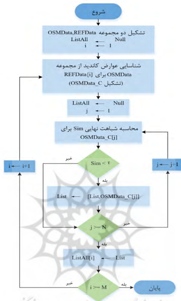
نگاره ۲: فلوجارت الگوریتم تناظریابی برای دو مجموعه داده رسمی و OSM
