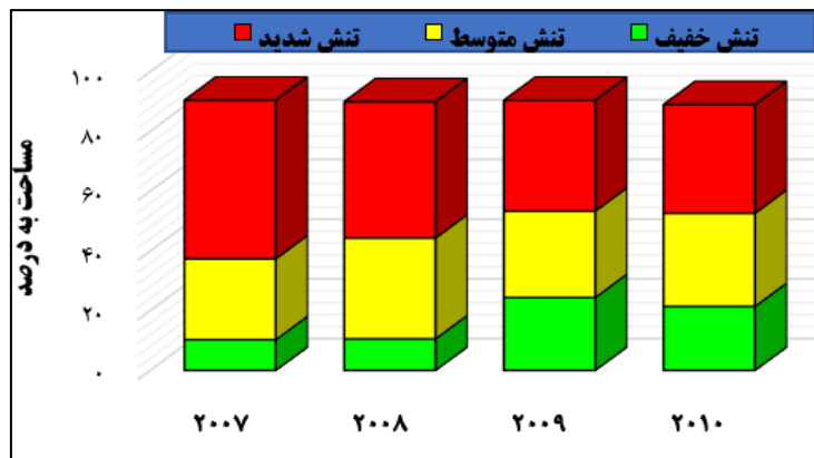
شکل (۱۳). منطقه کشاورزی در شرایط تنش خشکی WDI در روز ژولایوس ۱۵۳ برحسب درصد
