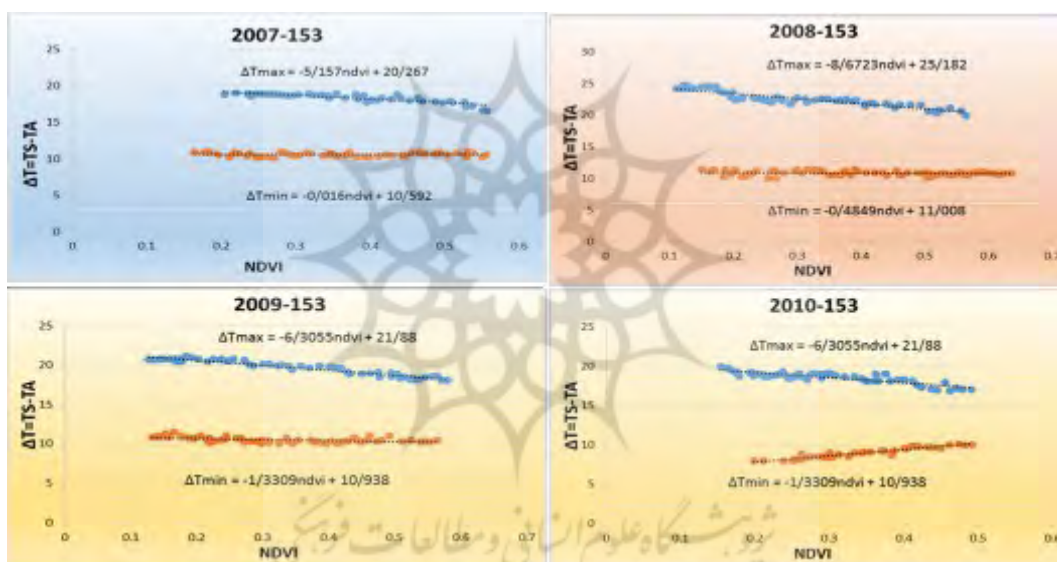
شکل (۸). لبه خشک و مرطوب از رابطه فضایی NDVI-ΔTS روز ژولایوسی ۱۵۳ در حوضه آبریز سیمینه رود (۲۰۱۰-۲۰۰۷)
