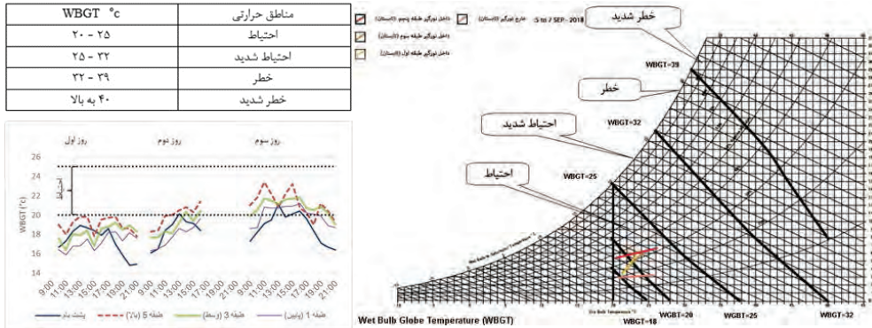
شکل ۸. راست: شاخص WBGT در طبقات و خارج نورگیر فصل تابستان ۱۳۹۷ بر روی نمودار سایکرومتریک، چپ بالا: مناطق حرارتی دمای تر کروی، چپ پایین: شاخص WBGT در طبقات و خارج نورگیر، چهاردهم تا شانزدهم شهریور ۱۳۹۷
