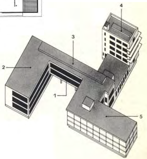
شکل ۶. مدرسه باهاوس در شهر دسا در آلمان منبع: Norwich, 1979, 237
