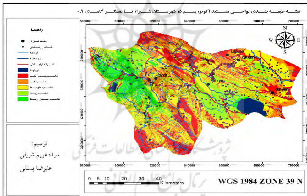
شکل ۱۴- نقشه طبقه بندی نواحی مستعد اکوتوریسم در شهرستان شیراز با استفاده از عملکرد گامای ۰/۹
