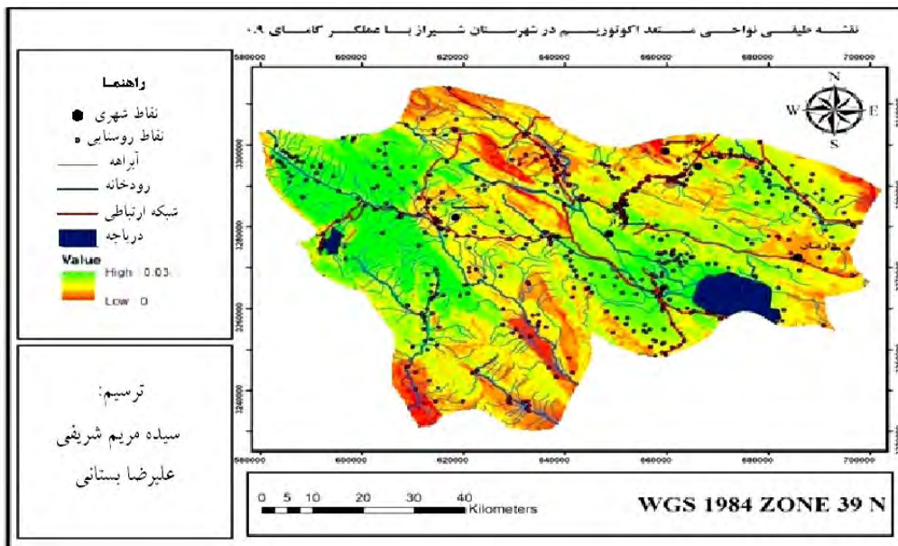
شکل ۱۳- نقشه طیفی نواحی مستعد اکوتوریسم در شهرستان شیراز با استفاده از عملکرد گامای ۰/۹
