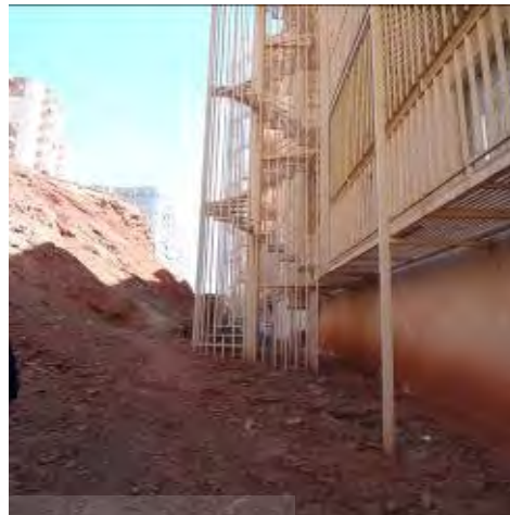
شکل ۷- نمونه‌ای از جریان‌ات گلی در پای دامنه که با حرکت به سمت مجتمع مسکونی به مرور زمان موجب دفن نیم طبقه‌ی اول مجتمع شده است
