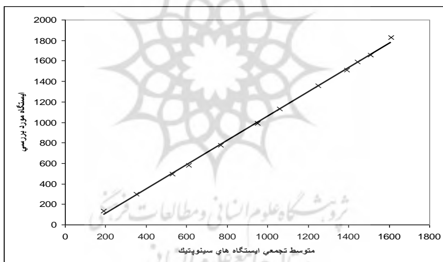
شکل ۱. منحنی جرم مضاعف برای ایستگاه باران‌سنجی بیرجند
