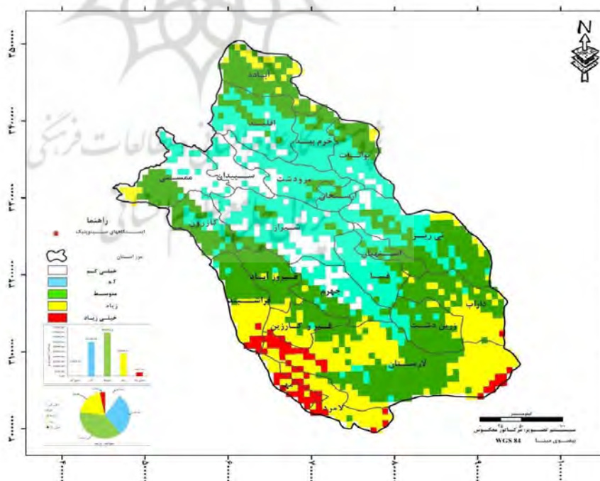
شکل ۳: نقشه وزن‌دهی کانون‌های گردوغبار به تفکیک شهرستان‌ها
