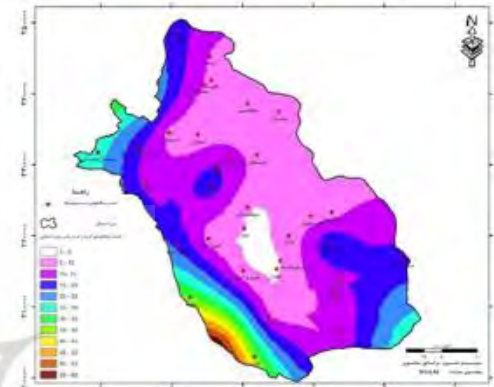
فراوانی توفان‌های گردوغبار در طی دوره زمانی (۱۳۸۰-۱۳۹۴)
