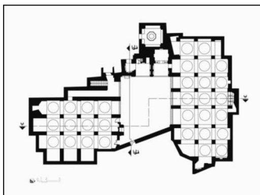
نقشه ۶: پلان مسجد فرط (میرخلیلی، ۱۳۹۰: ۴۸)
