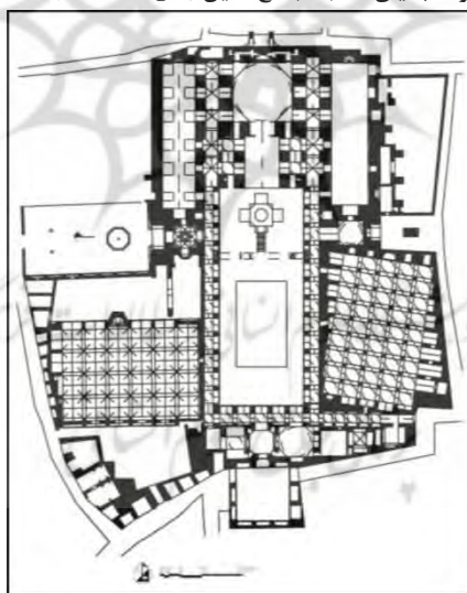
نقشه ۵: پلان مسجد جامع (آرشیو اداره کل میراث فرهنگی، صنایع دستی و گردشگری استان یزد)
