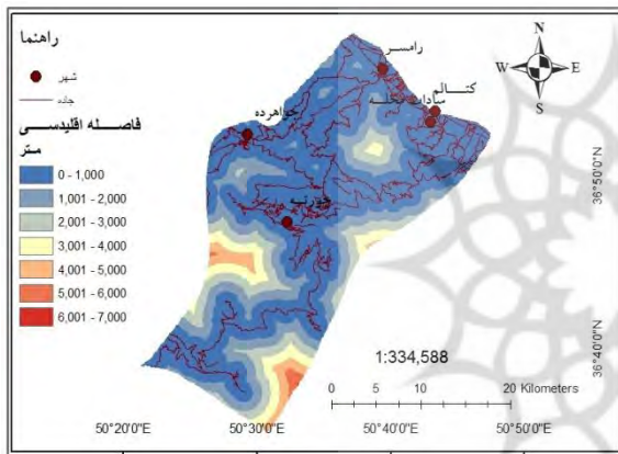
شکل ۵: برآورد فاصله اقلیدسی از راهها
