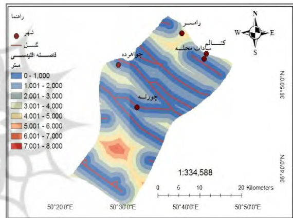
شکل ۴: برآورد فاصله اقلیدسی از گسل ها
