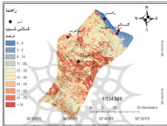
شکل ۴: کلاس شیب شهرستان
