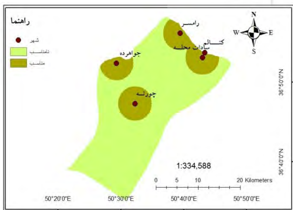
شکل ۳: پهنه‌های مناسب و نامناسب شهری
