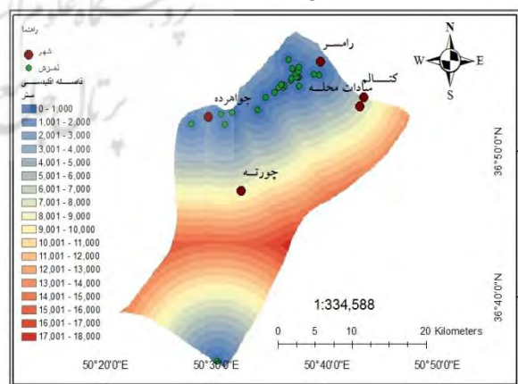
شکل ۶: برآورد فاصله اقلیدسی از پهنه‌های لغزشی
