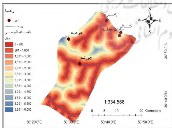
شکل ۷: برآورد فاصله اقلیدسی از رودخانه‌ها
