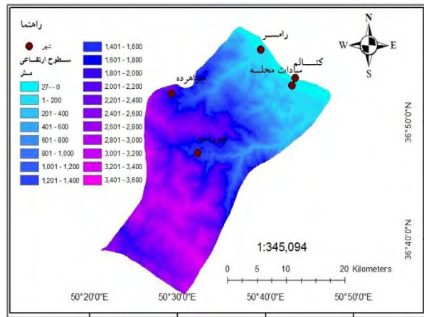
شکل ۲: سطوح ارتفاعی شهرستان
