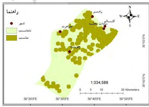
شکل ۲: پهنه‌های مناسب و نامناسب روستایی
