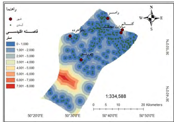
شکل ۲: برآورد فاصله اقلیدسی از آبادیها
