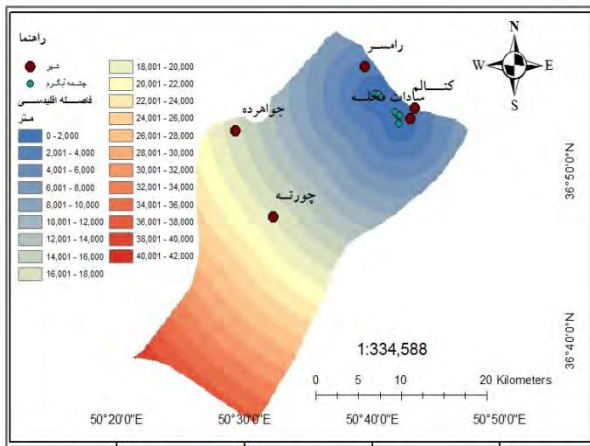
شکل ۳: برآورد فاصله اقلیدسی از چشمه‌های آبگرم
