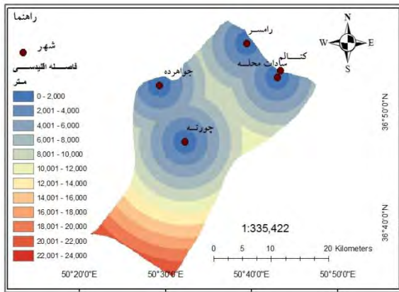
شکل ۳: برآورد فاصله اقلیدسی از مراکز شهری
