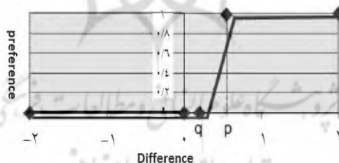
شکل ۳: مثالی از یک معیار تعمیم یافته
