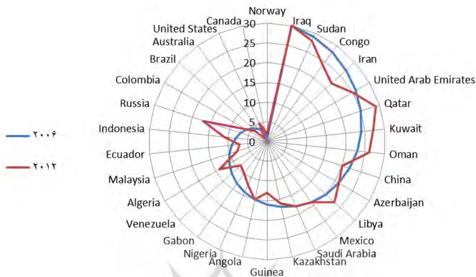
شکل ۴: نمودار رتبه کشورها در سال‌های ۲۰۰۶ و ۲۰۱۲
