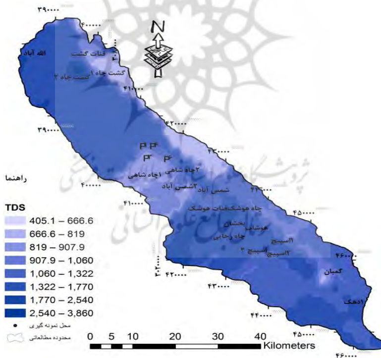
شکل ۵. پراکنش مواد جامد محلول در آب (TDS)
