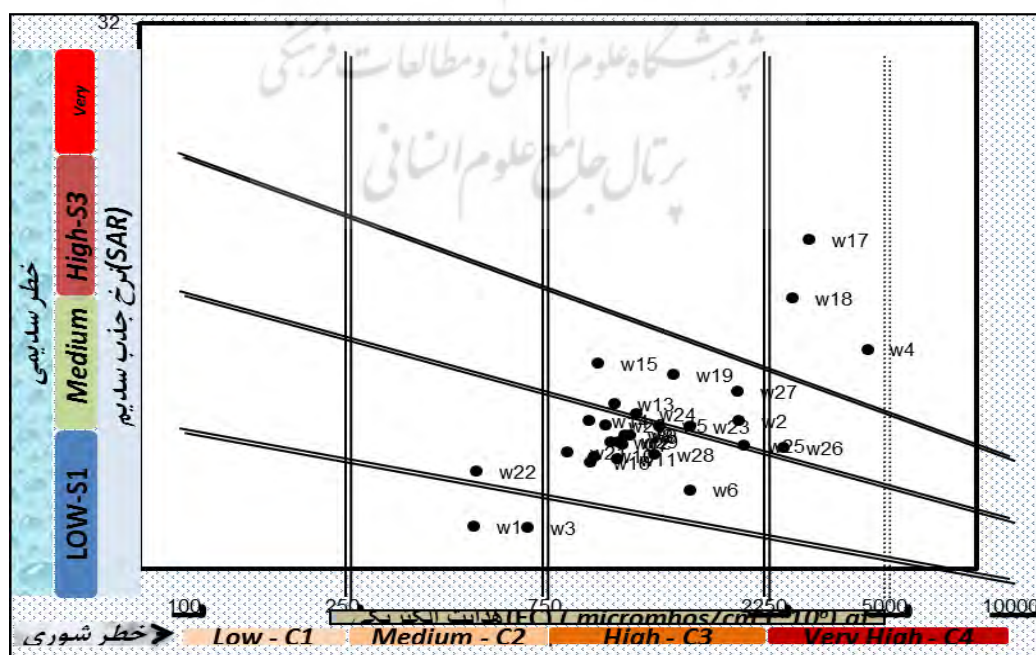
شکل ۱۲. نمودار ویلکوکس نمونه‌های آب زیرزمینی دشت سراوان
