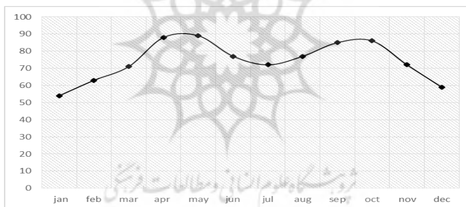
شکل ۴: نمودار شاخص اقلیم گردشگری TCI در ماه‌های مختلف طی سال‌های ۲۰۱۰ - ۱۹۵۱
