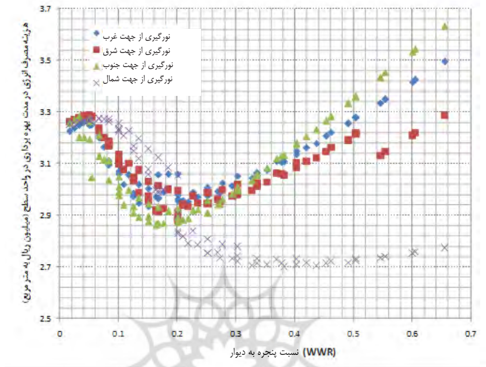
شکل ۳. هزینه مصرف انرژی در مدت بهره‌برداری از کلاس استاندارد واقع در شیراز
