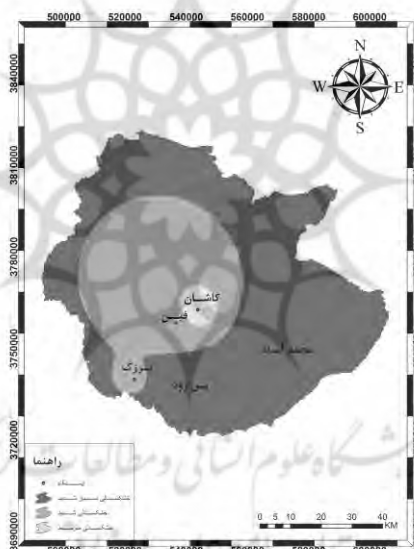
شکل (۴) نقشه‌ی وضعیت خشکسالی درمقیاس زمانی ۶ ماهه در دشت کاشان.
