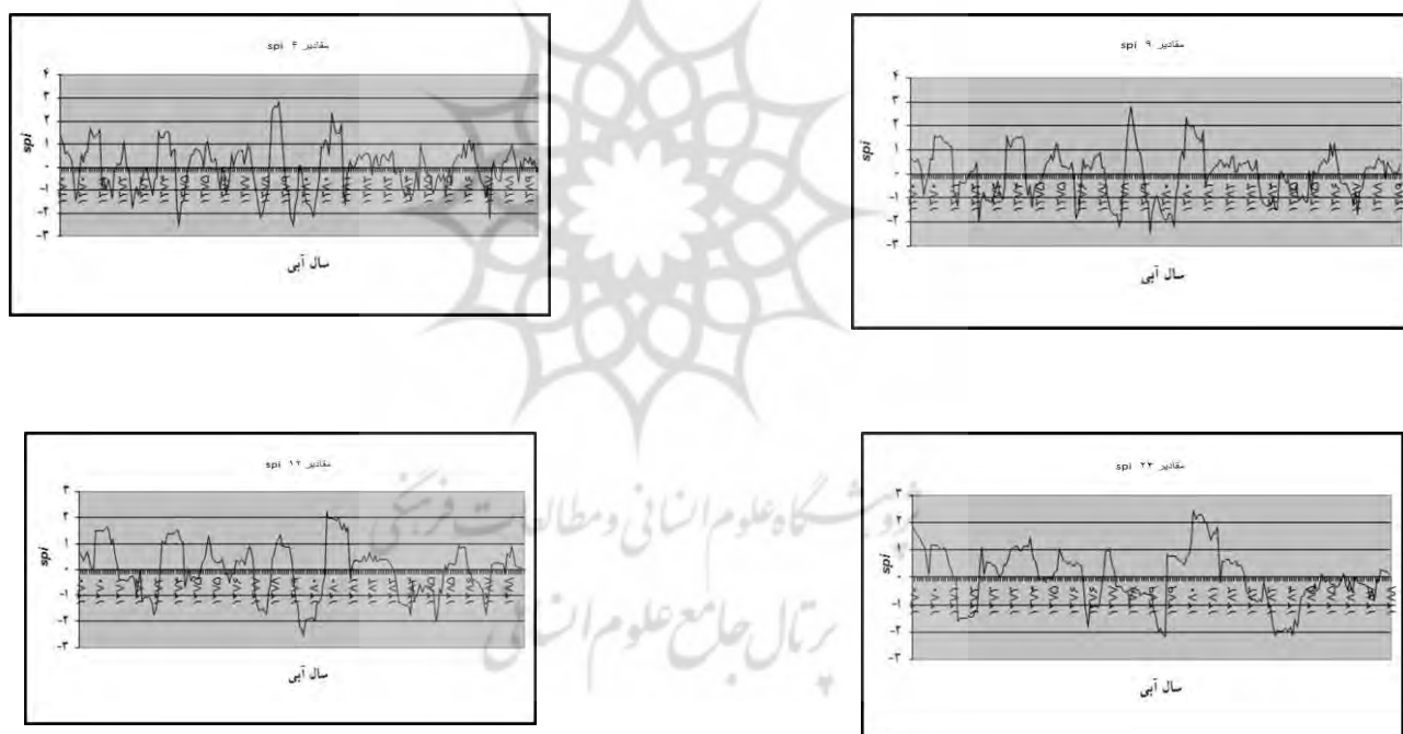
شکل (۲) نمودار خشکسالی‌ها و ترسالی‌های ایستگاه کاشان (نمونه) در مقیاس‌های زمانی مورد مطالعه (۶،۹،۱۲ و ۲۴ ماهه)
