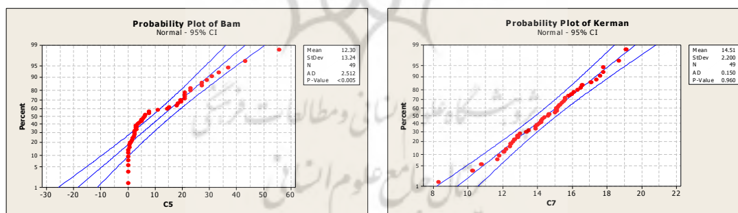
شکل ۳- نمونه ای از توزیع غیرنرمال داده ها
