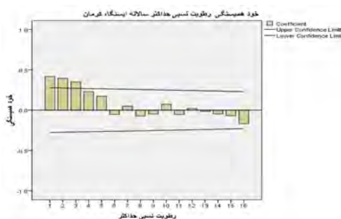
شکل ۱۳- رطوبت نسبی حداکثر سالانه ایستگاه کرمان
