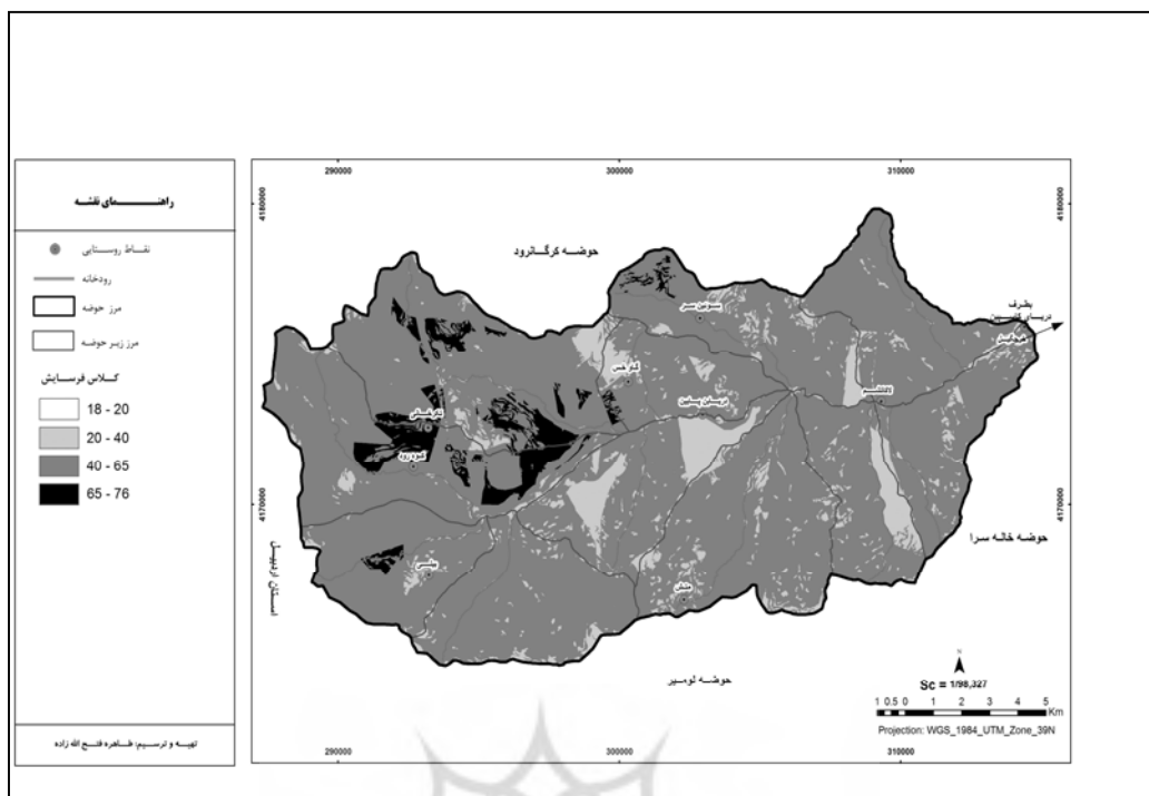
شکل ۲: نقشه فرسایش حوضه آبخیز ناورود به روش FAO
