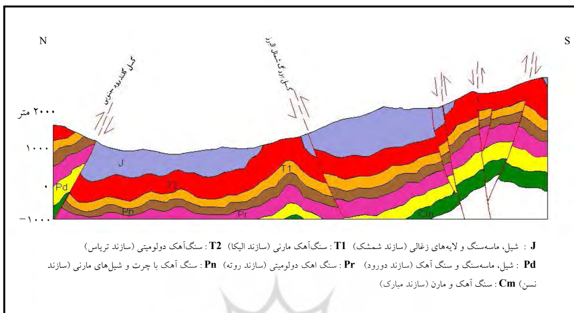
شکل ۲: نیمرخ زمین شناسی حوضه آبریز لایویج رود ( مأخذ: نقشه زمین شناسی ۱:۱۰۰۰۰۰ آمل) منبع: نگارندگان
