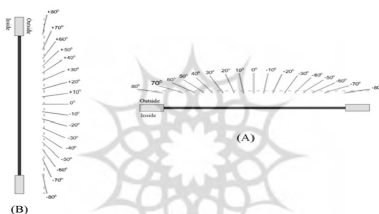
تصویر ۳. حالات شبیه‌سازی شده برای لوورهای عمودی در جبهه شرق و غرب (A) و برای لوورهای افقی در جبهه جنوب ساختمان (B)
