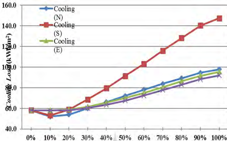
تصویر ۱. میزان بار سرمایش سالانه ساختمان با درصد پنجره‌های مختلف در جبهه‌های مختلف ساختمان برای شیراز
