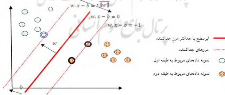
شکل ۱- ساختار مدل طبقه‌بندی ماشین بردار پشتیبان
