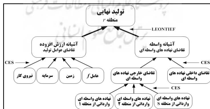
شکل (۵): ساختار تکنولوژی بنگاه در مدل GTAP
