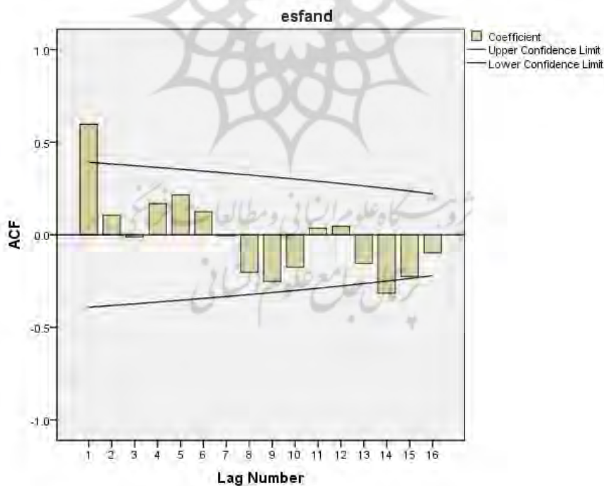
شکل ۱۲) نمودار تابع خودهمبستگی دمایی حداکثر مطلق اسفندماه در ایستگاه کیش
