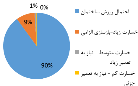
شکل ۹: درصد و میزان خسارت مدارس در زلزله‌هایی با شدت MSK9
