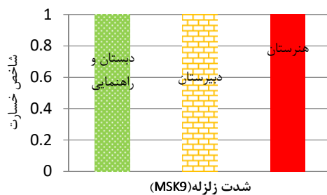
شکل ۶: متوسط شاخص خسارت در زلزله‌هایی با شدت MSK9
