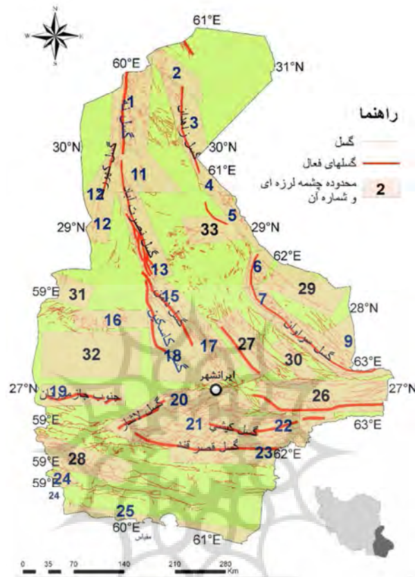
شکل ۲: موقعیت گسل‌های استان سیستان و بلوچستان و بلوچستان (پرتابیان و همکاران ۱۳۹۵)
