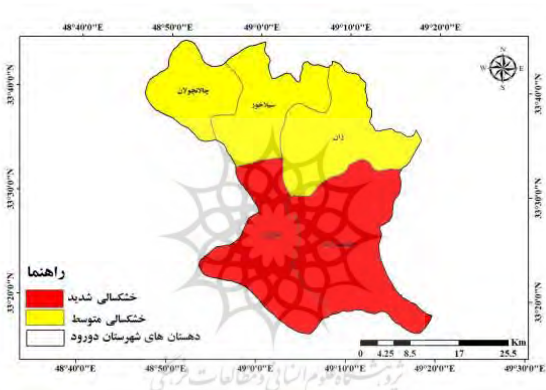
شکل ۳. وضعیت خشکسالی در دهستان‌های مطالعه شده براساس شاخص SPI
