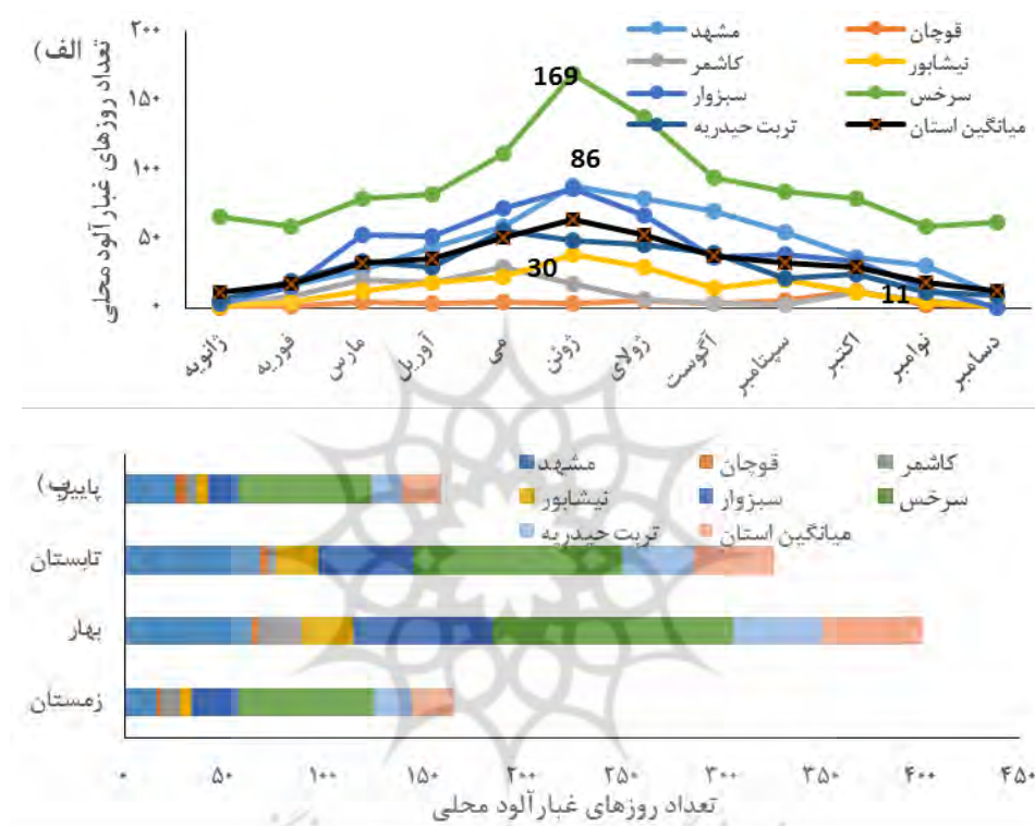
شکل ۳. میانگین ماهیانه و فصلی روزهای غبارآلود محلی در ایستگاه‌های استان طی دوره آماری ۱۹۹۰ - ۲۰۱۶
