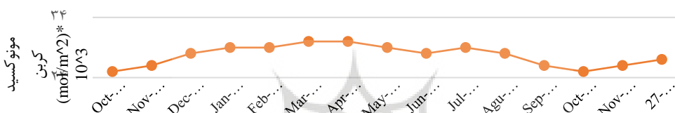
شکل ۳: نمودار تغییرات میانگین ماهانه آلاینده CO در طول ۲۰۱۸-۲۰۱۹
