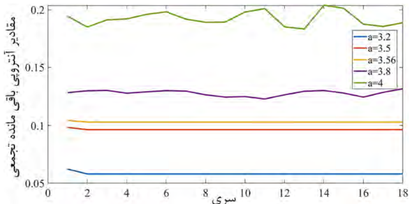
شکل ۱: تشخیص بحران به وسیله معیار آنروپی باقی مانده تجمعی در حالت نظری با استفاده از نقشه لوجستیک
