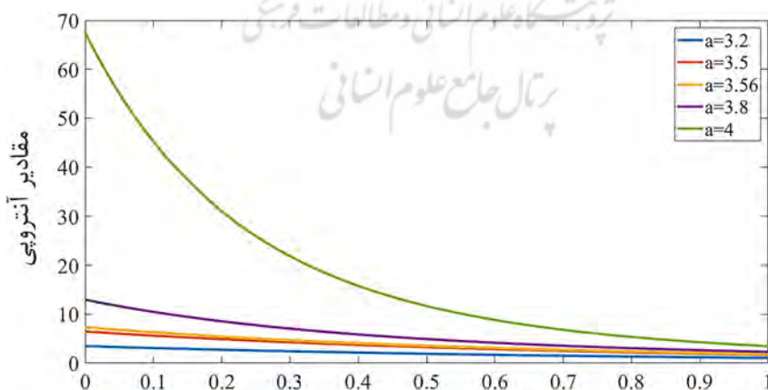
شکل ۲: مقدار آنروپی باقی مانده تجمعی فراکتالی برای پنج سری ساختگی به وسیله نقشه لوجستیک در درجات فراکتالی مختلف
