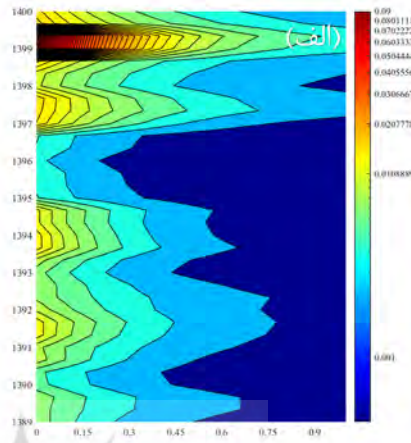
شکل ۳: (الف) کانتور آنتروپی باقی مانده تجمعی فراکتالی برای سری شاخص کل به منظور مقایسه قدرت پیش بینی بحران دو معیار پیشنهادی؛ (ب) شاخص کل، حجم معاملات، ارزش معاملات، و قیمت دلار
