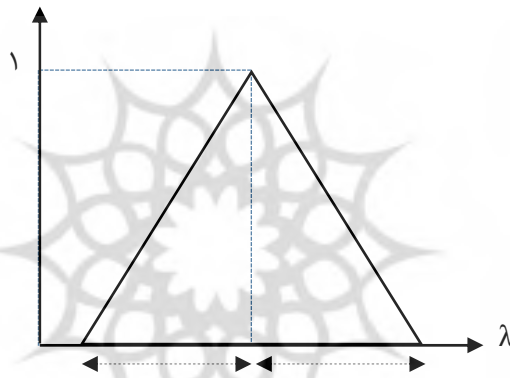
شکل ۱. عدد فازی مثلثی و پارامترهای آن
